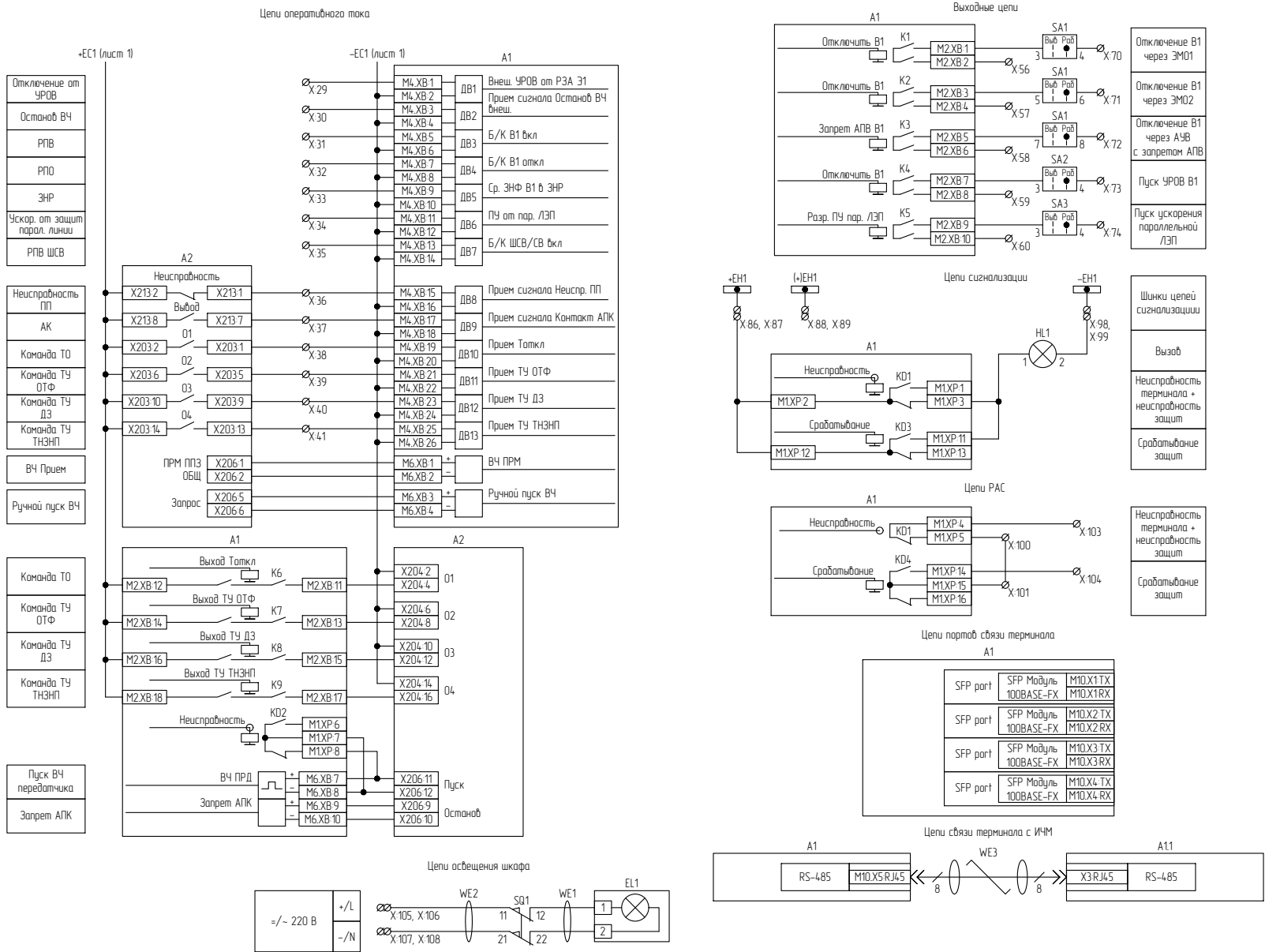
Рисунок В.2 – Схема электрическая принципиальная (часть 2)
